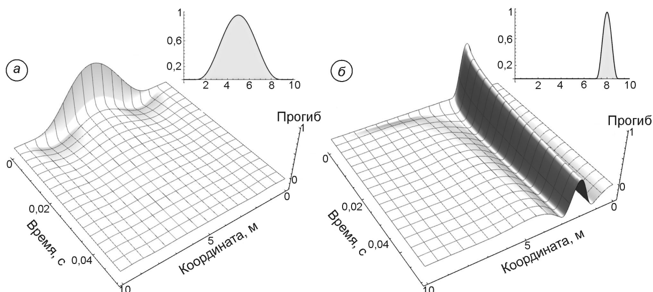
Рис. 7. Эволюция прогибов при возмущениях на интервалах различной протяжённости: а – 70%; б – 10% ширины пластины
