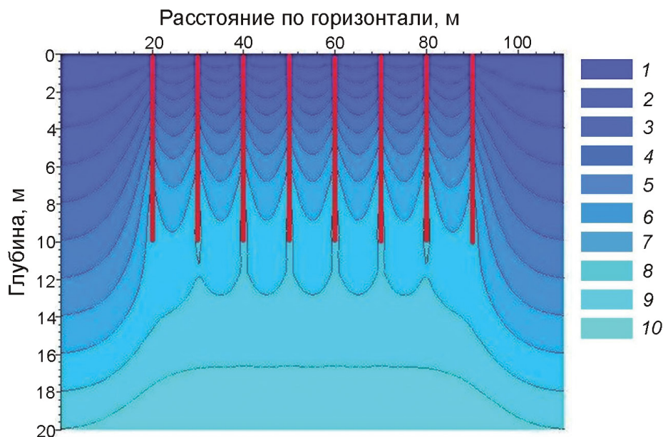
Рис. 2. Температурное поле в леднике в конце годового периода льдообразования в трещинах при начальной температуре на глубине основания активного слоя ледника -2^\circ\text{C} и начальной толщине нижележащего холодного слоя 20 м.
