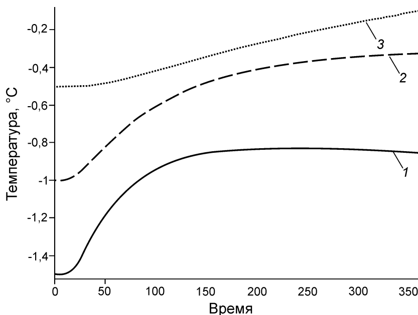
Рис. 5. Годовая динамика температуры в центральной части области трещиноватости на различных глубинах при начальной температуре основания активного слоя -2^{\circ}\text{C} и начальной толщине холодного слоя 20 м:
