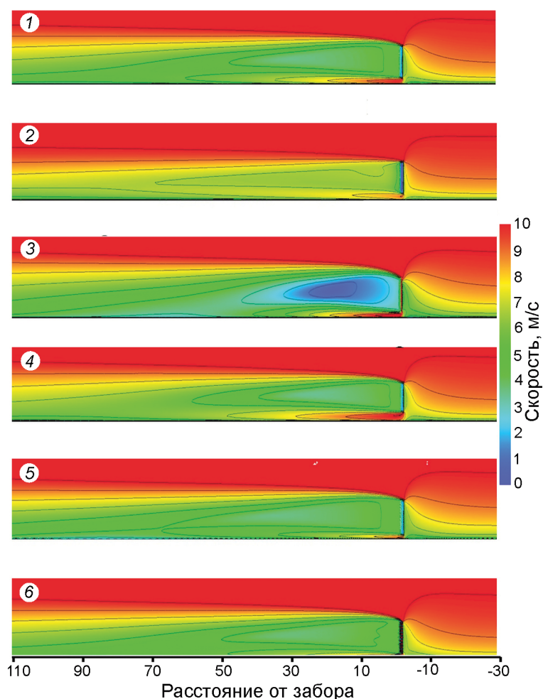
Рис. 3. Магнитуа поля скорости в вертикальном сечении для разных вариантов (см. таблицу), м/с.
