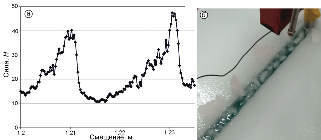
Рис. 4. Прорезание ледяного поля вертикальным индентором:
