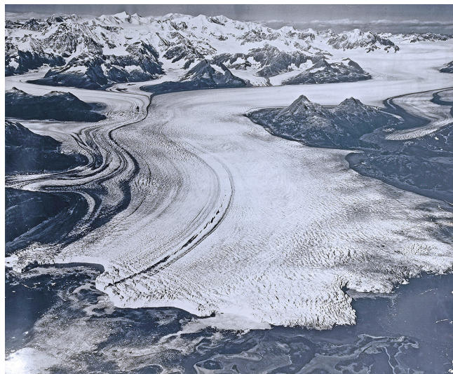
Рис. 1. Ледник Колумбия в 1970 г.
