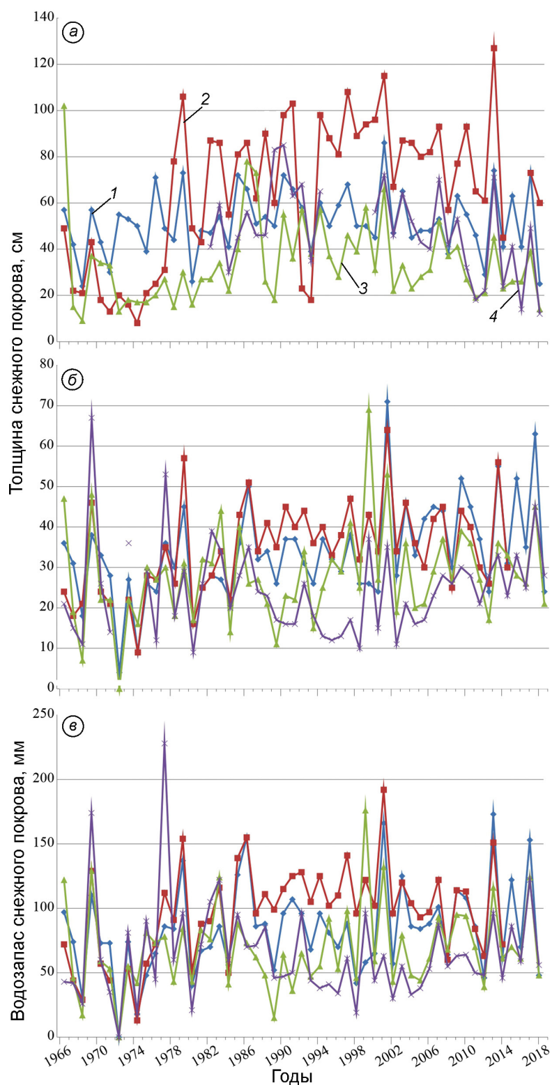
Рис. 3. Толщина снежного покрова на метеоплощадках (а) и маршрутах (поле) (б), водозапас снежного покрова на маршрутах (поле) (в) на период максимума по данным ГМС:
