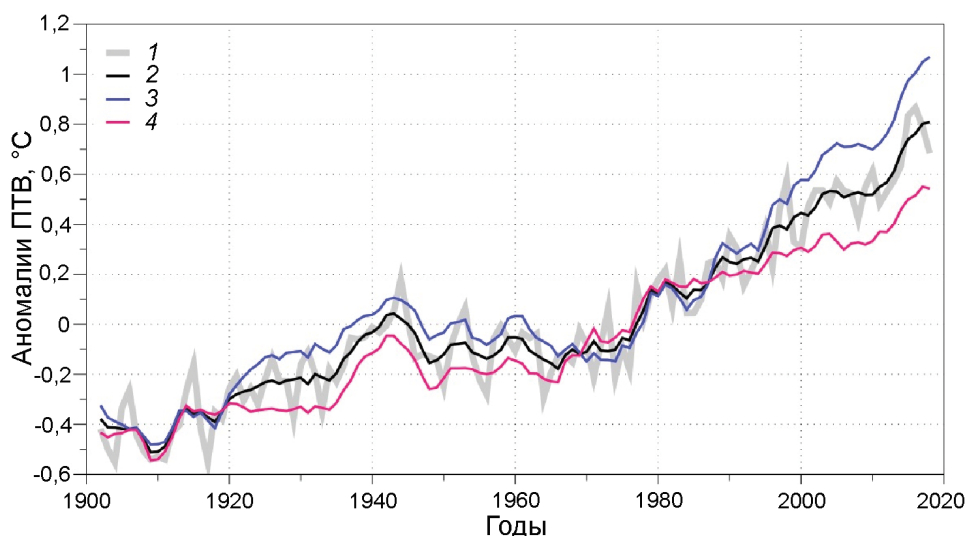
Рис. 2. Аномалии среднегодовой приземной температуры воздуха (°C) в период 1900–2015 гг.:
