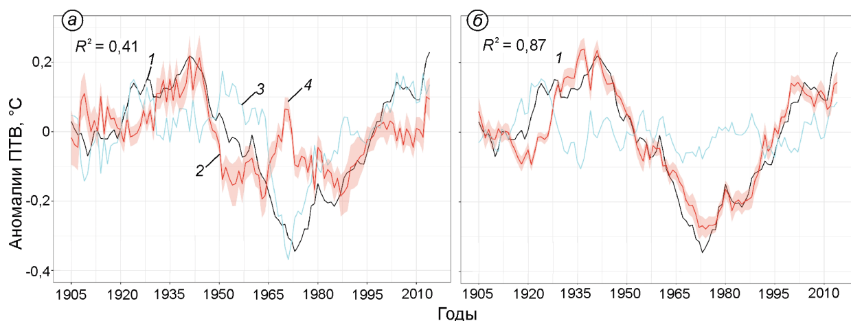
Рис. 9. Многолетние изменения зимней (январь–март) приземной температуры воздуха (°C) в Северном полушарии по данным наблюдений HadCRUT5.0 (Morice et al., 2021) и рассчитанные с применением множественной регрессии наблюденной приземной температуры воздуха на индексы:
