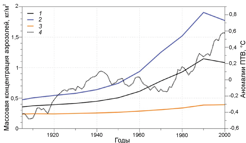
Рис. 6. Массовая концентрация аэрозолей ( \text{кг}/\text{м}^2 ) по данным климатической модели GISS для CMIP5 с заданной реконструкцией эмиссий антропогенных аэрозолей:
