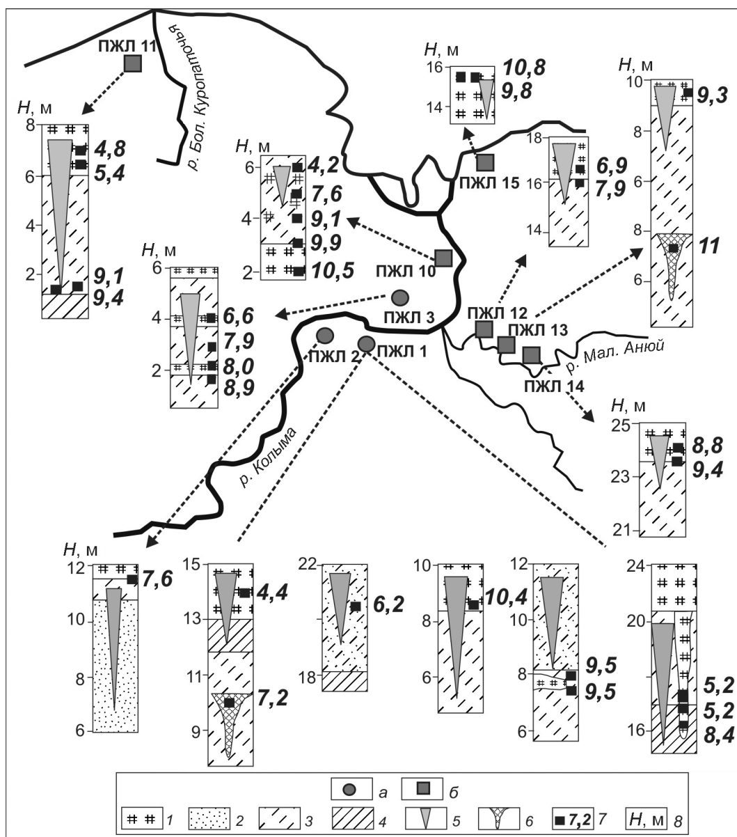
Рис. 3. Стратиграфия и ^{14}\text{C} датировки отложений аласов с повторно-жильными льдами (ПЖЛ) в низовьях р. Колыма по материалам авторов (а) и ранее опубликованным данным (б) (более подробная информация о датировках приведена в табл. 1).
