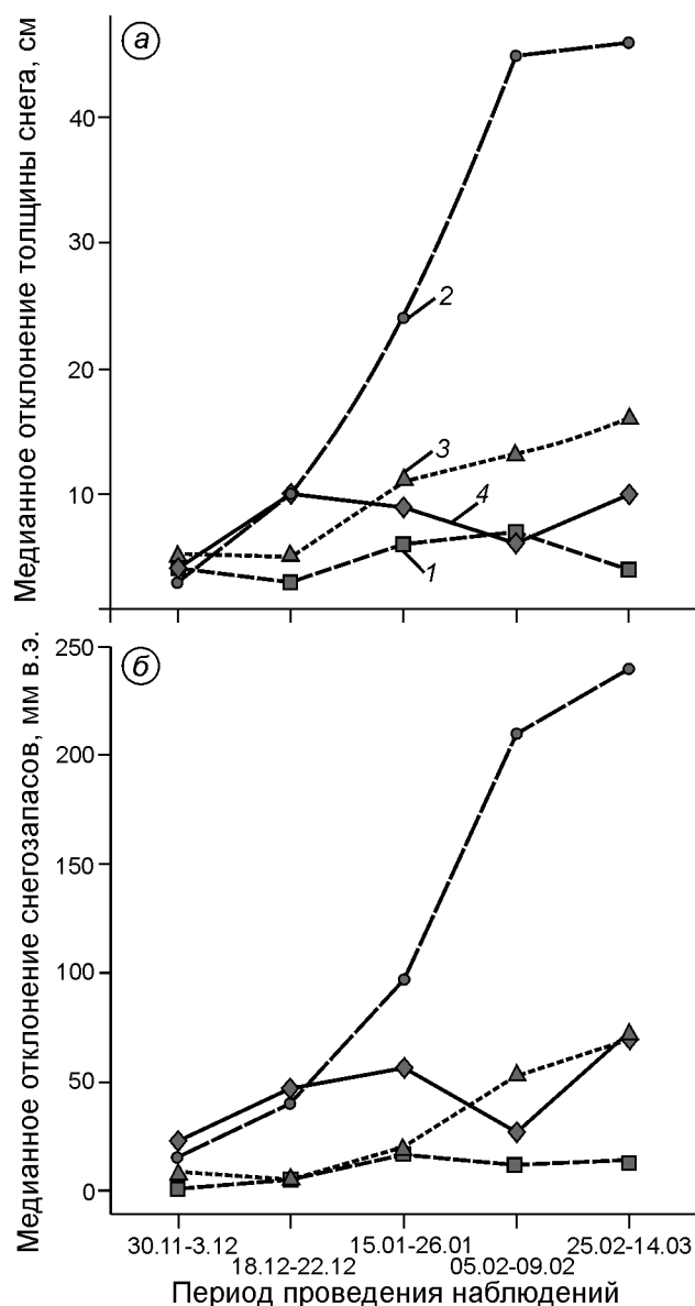
Рис. 4. Медианное абсолютное отклонение толщины снежного покрова (а) и снегозапасов (б) по данным измерений по стационарной рейке и маршрута метеостанции (при наличии) относительно бассейновых наблюдений за тот же период в течение зимы 2019/20 г.:
