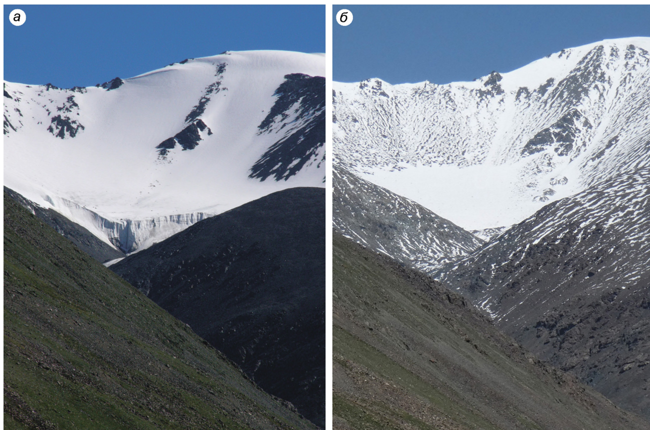
Рис. 4. Вид ледника № 15 через 16 лет и 31 год после сейсмособытия 1988 г.
