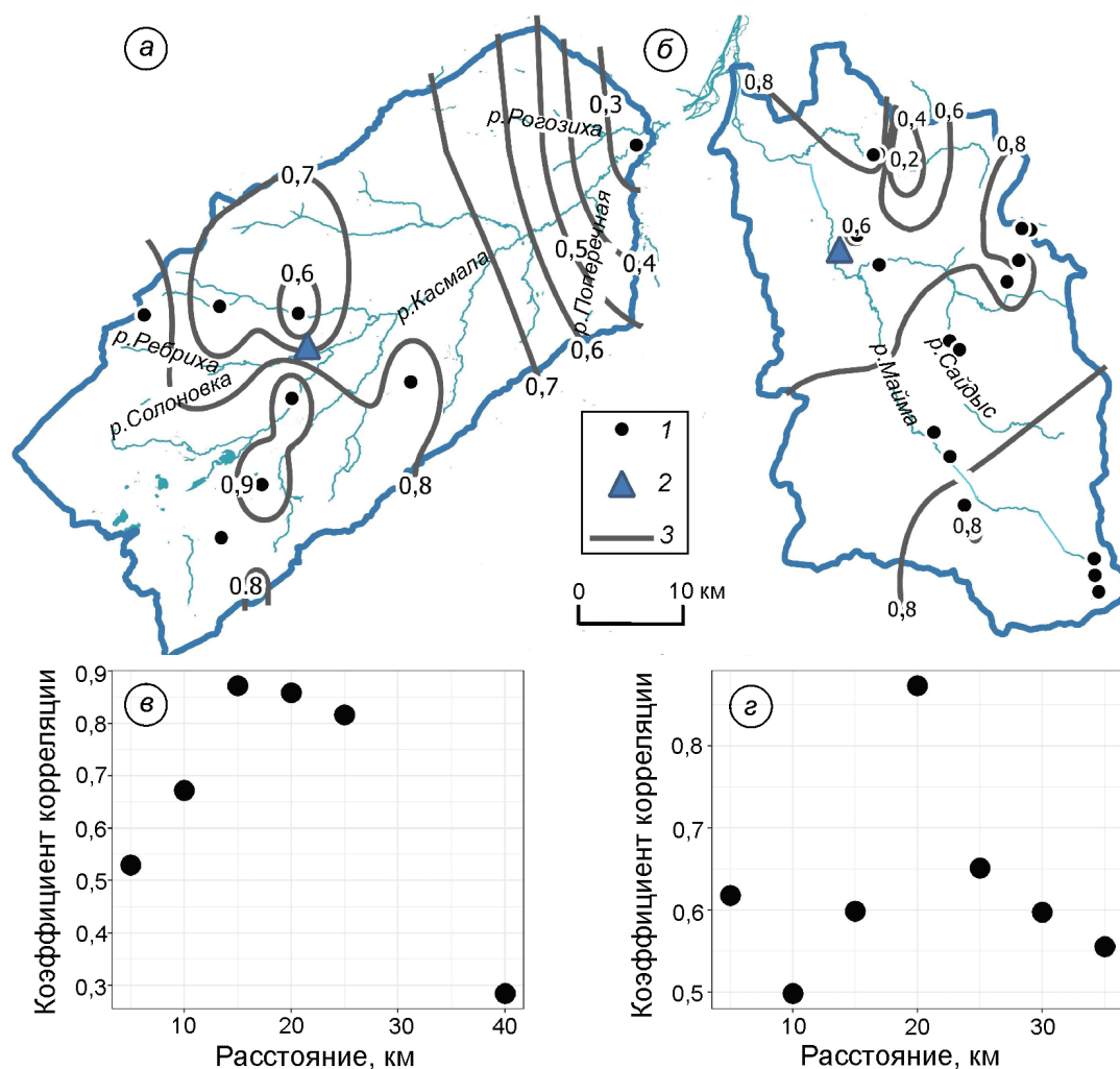
Рис. 6. Пространственная дифференциация коэффициентов корреляции и графики корреляционных функций в бассейнах рек Касмала (а, в) и Майма (б, г):
