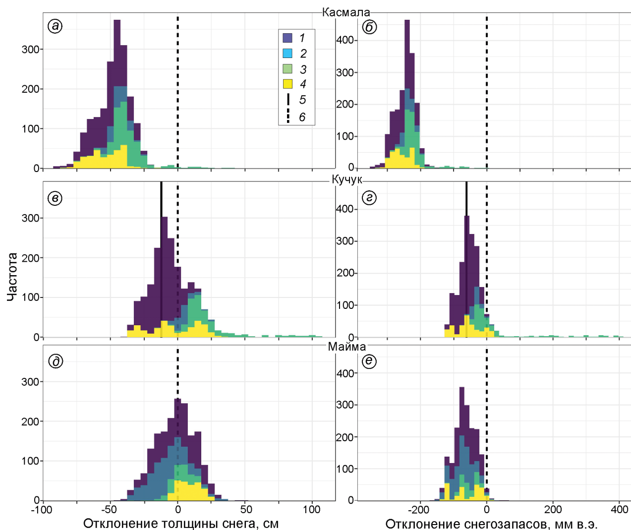
Рис. 5. Распределение значений отклонений толщины снежного покрова и снегозапасов в различных природных комплексах бассейнов рек Касмалы (а, б), Кучука (в, г) и Маймы (д, е) в период максимума снегонакопления относительно наблюдений на метеостанциях за тот же временной период в 2019/20 г.:
