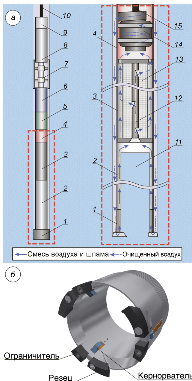
Рис. 3. Предлагаемый способ колонкового механического бурения.
