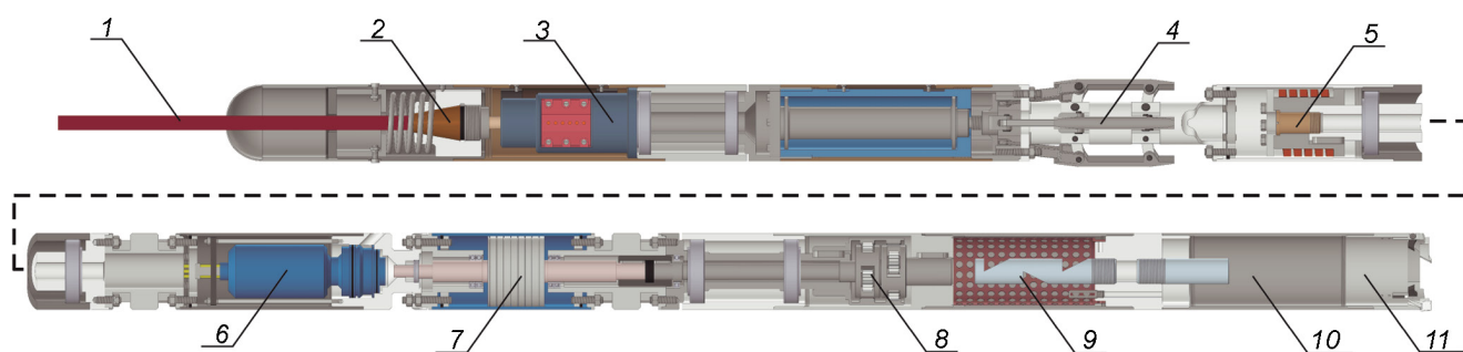
Рис. 2. Буровой снаряд КЭМС-127 (колонковая труба и шламособорный отсек – не в масштабе):
