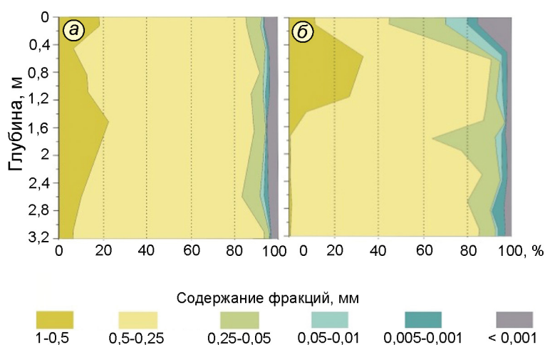
Рис. 3. Изменение гранулометрического состава с глубиной:
