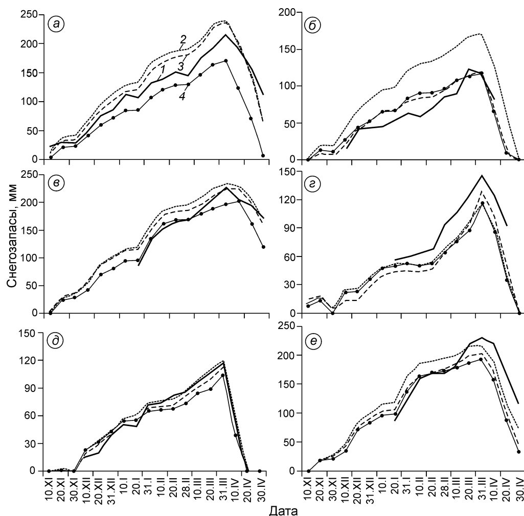
Рис. 4. Сопоставление расчётного и фактического снегозапаса по отдельным снегомерным маршрутам: а – Чердынь (поле); б – Кудымкар (поле); в – Усть-Черная (лес); г – Октябрьский (лес); д – Бол. Соснова (поле); е – Нагорское (лес); 1 – данные снегомерных съёмок; 2 – модель GEM; 3 – модель GFS; 4 – модель ПЛ-АВ
