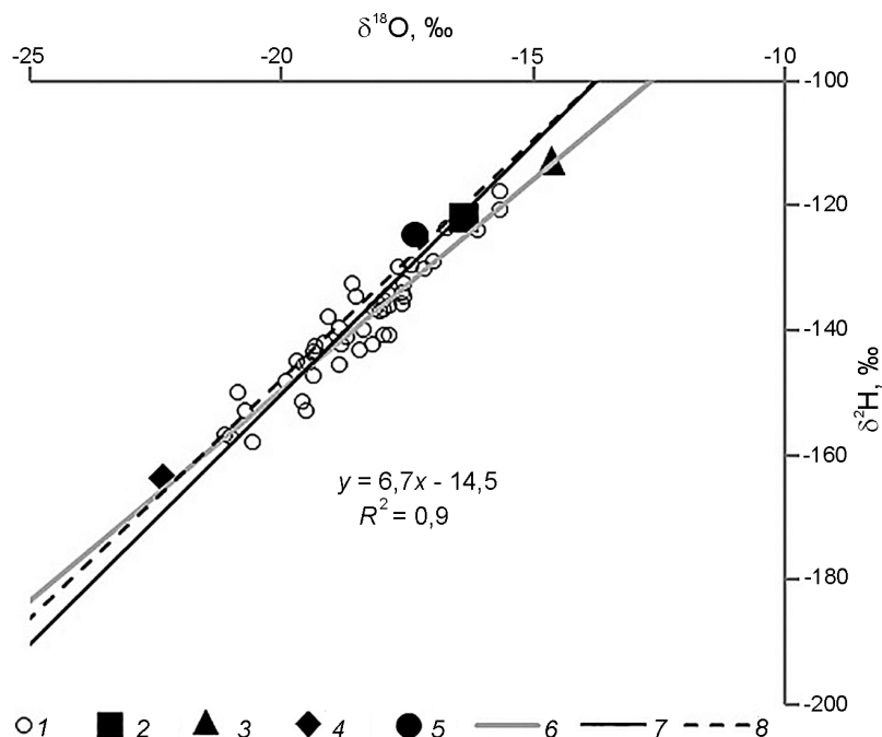
Рис. 3. Содержание \delta^2\text{H} и \delta^{18}\text{O} в снеге по данным валовых проб из снежной толщи в марте 2016 г. (1) и среднемесячный изотопный состав зимних атмосферных осадков в г. Петрозаводск:
