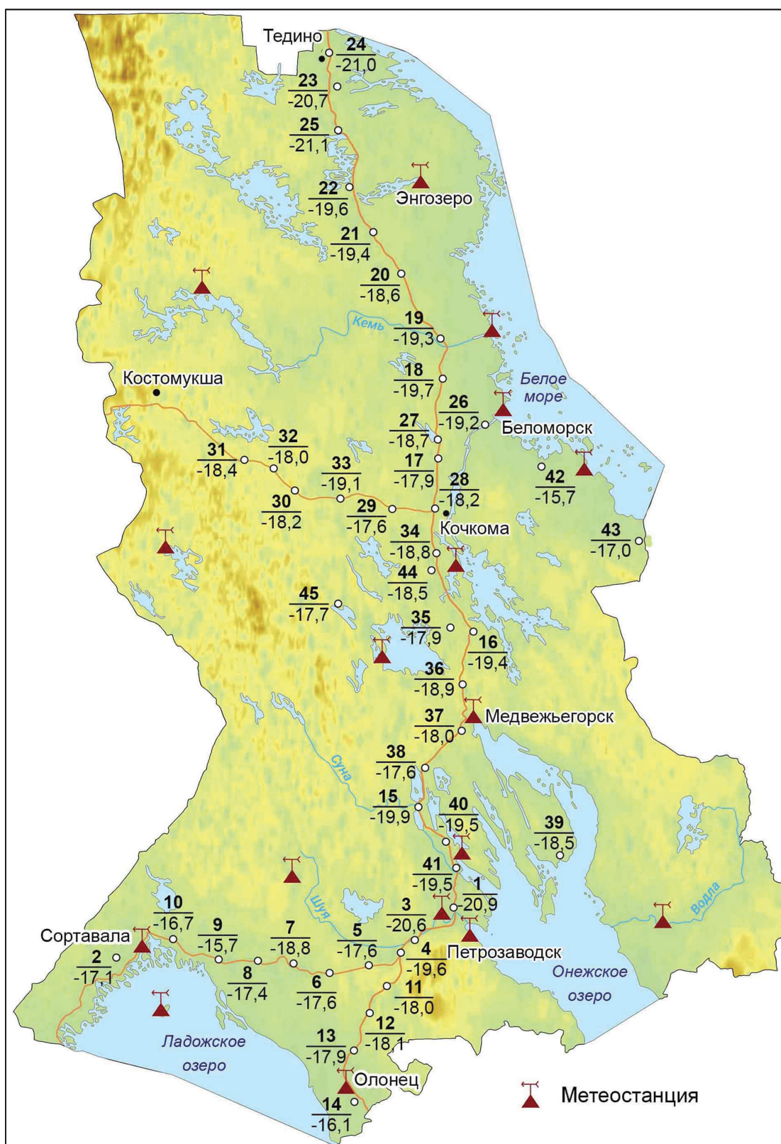
Рис. 1. Расположение пунктов отбора образцов снега и значения \delta^{18}\text{O} на территории Карелии.
