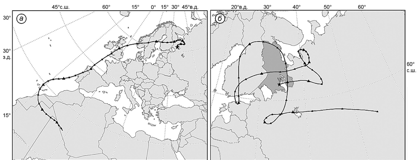
Рис. 4. Обратные траектории движения воздушных масс (использован онлайн инструмент HYSPLIT на сайте NOAA [23]), вызывающие осадки на территории Карелии 24.12.2015 г. (а) и 13.01.2016 г. (б).
