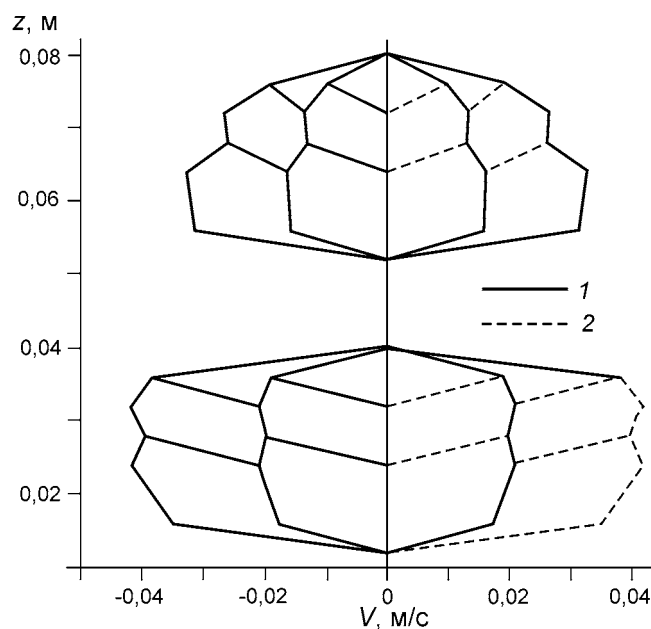
Рис. 4. Распределения по вертикали поперечных скоростей потока: 1 – на разрезе, соответствующем входу в талик; 2 – на разрезе, соответствующем выходу из талика
