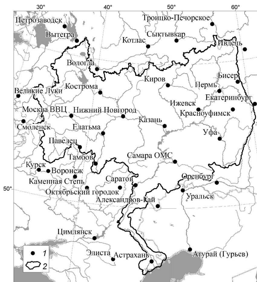
Рис. 1. Расположение метеорологических станций, данные наблюдений которых использованы для апробации модели:
