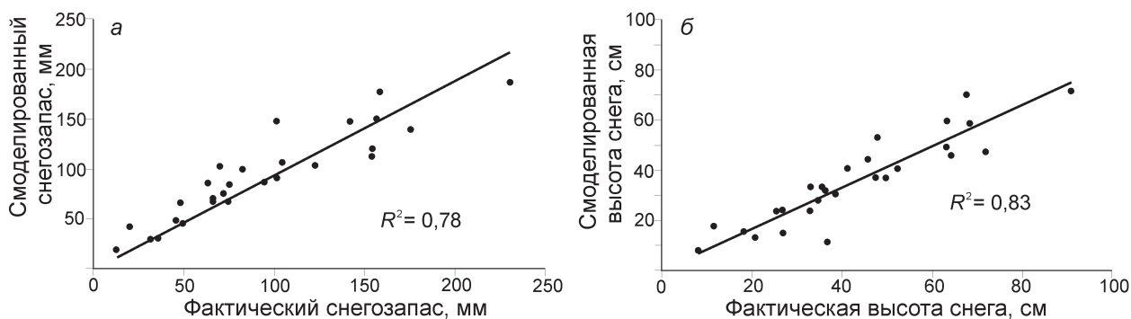
Рис. 5. Связь фактических и рассчитанных среднемноголетних максимальных снегозапасов (а) и максимальной в году высоты снега (б)
