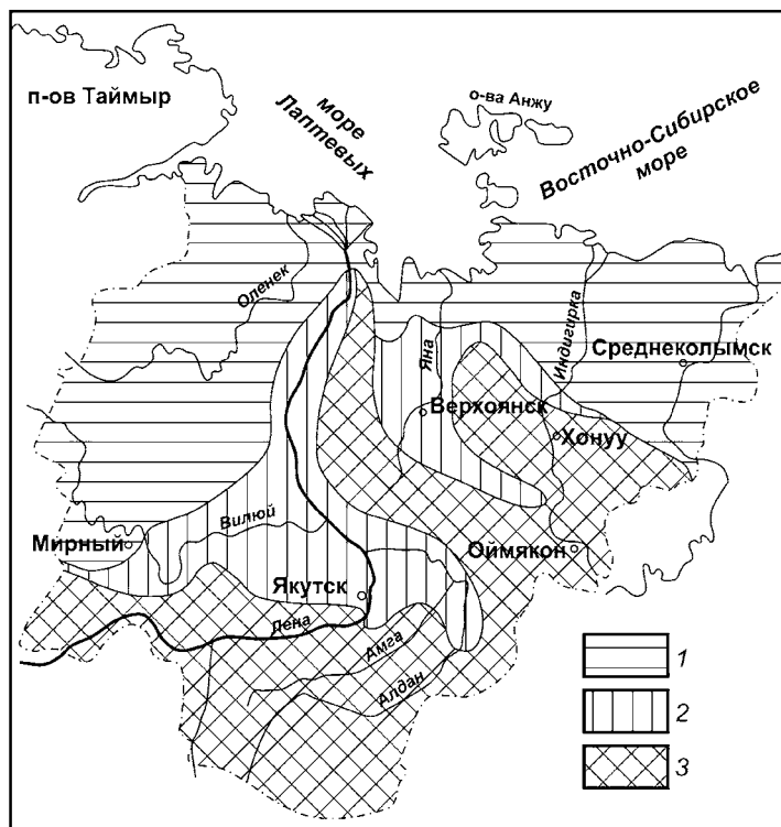
Рис. 2. Схема относительной наледности для территории Якутии:
