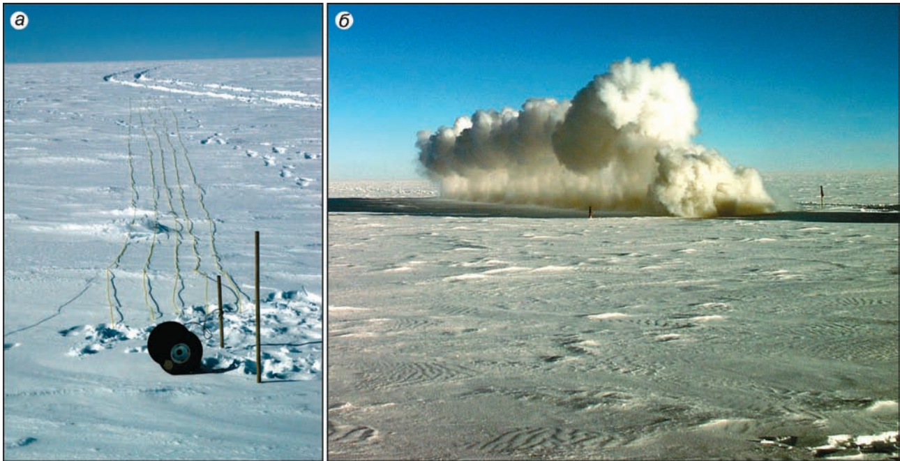
Рис. 3. Фотографии, на которых показано расположение линий детонирующего шнура (а) и возбуждение акустических волн (б) Fig. 3. Photos of the detonating cord position (а) and acoustic wave generation (б)
