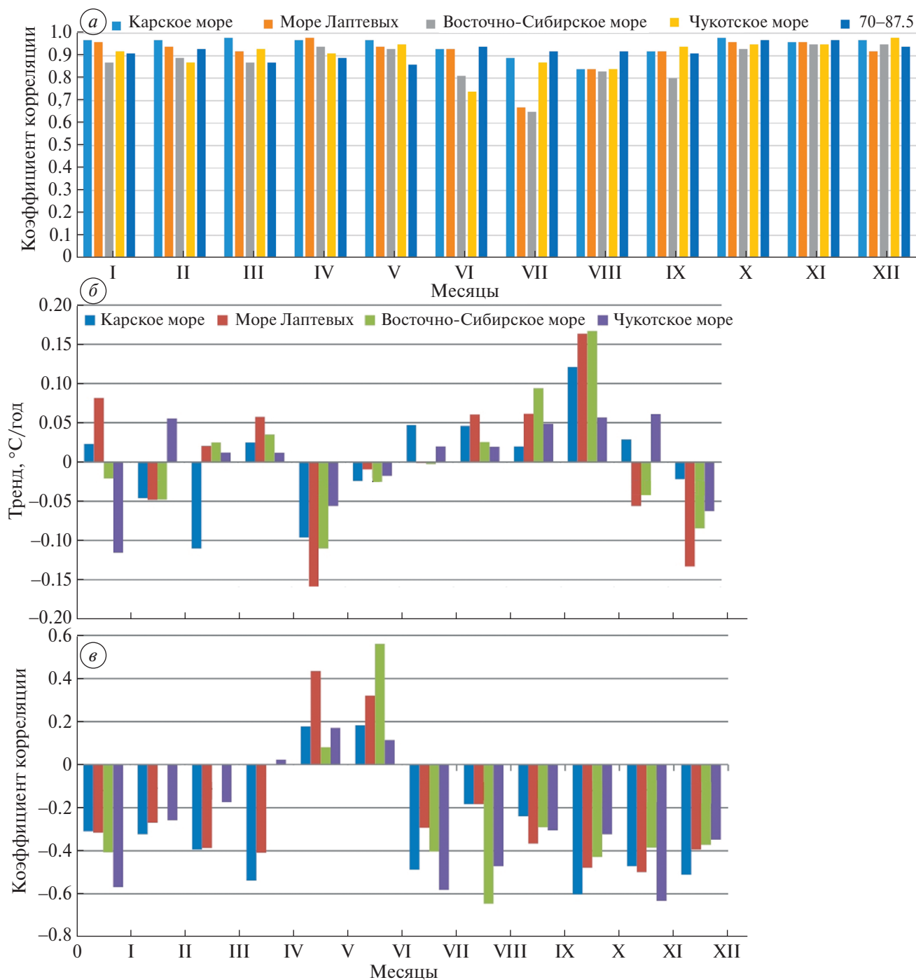
Рис. 4. Характеристики изменчивости температуры воздуха над акваториями морей Северного морского пути по реанализу ERA5 и корреляции между приращениями температуры и ледовитости для сравнения с расчётами, использующими температуру на метеостанциях: а – коэффициенты корреляции между средними температурами; б – коэффициенты тренда междумесечных приращений температуры по ERA5; в – коэффициенты корреляции между приращениями температуры по ERA5 и ледовитости.
