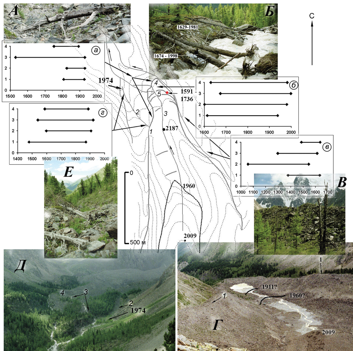
Рис. 6. Ледник и предполя левостороннего истока р. Шавла, местоположение и возраст образцов древесины:
