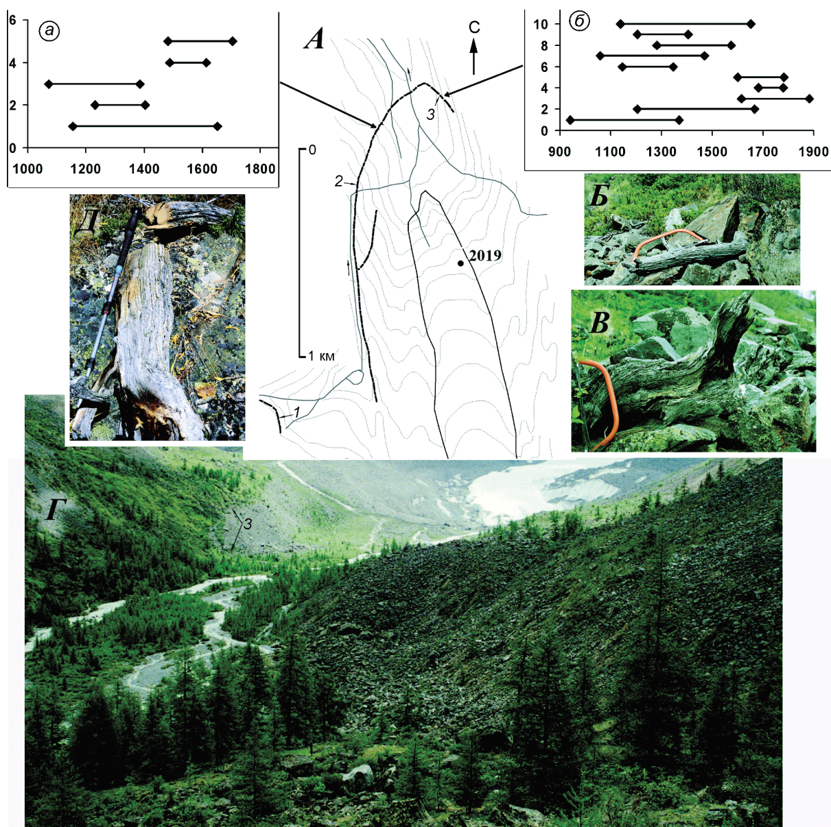
Рис. 5. Язык и предполя ледника Маашей, места отбора образцов на дендрохронологический анализ:
