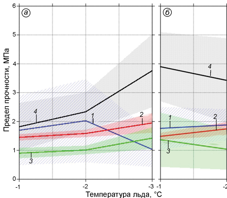
Рис. 4. Зависимость прочности морского льда на одноосное сжатие (МПа) от температуры (°C):
