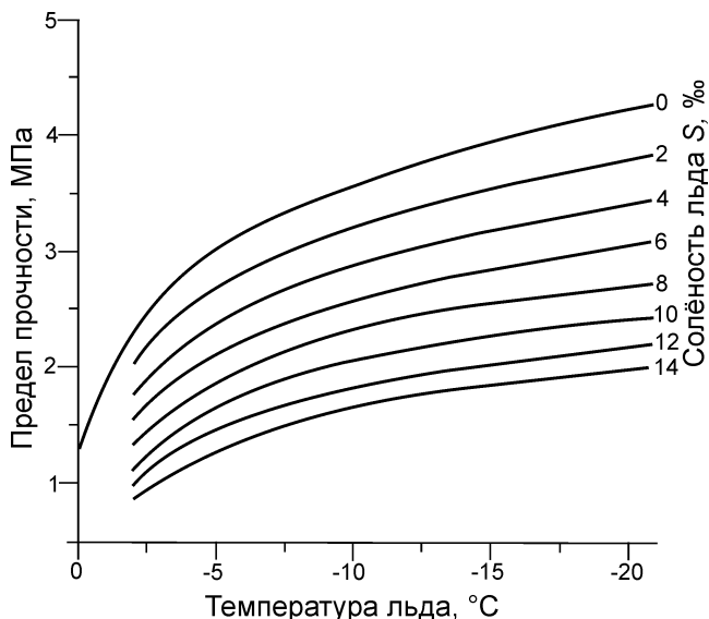
Рис. 3. Зависимости прочности льда на одноосное сжатие (МПа) от температуры (°C) при разной солёности льда (‰), построенные с использованием предрасчитанных полиномиальных функций по алгоритму В.В. Богородского [11]
