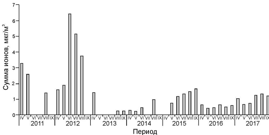
Рис. 1. Изменение суммарного содержания ионов в составе аэрозоля (апрель–сентябрь, 2011–2017 гг.) Fig. 1. Change of sum of ions in aerosol composition (April–September, 2011–2017)
