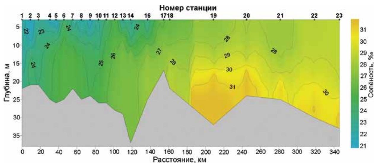
Рис. 2. Распределение солёности (‰) морской воды на океанографическом разрезе в Хатангском заливе и на выходе из него в море Лаптевых по данным экспедиции «Кара-лето–2016»
