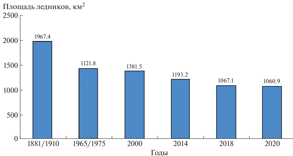
Рис. 2. Сокращение площади ледников Кавказа за 1881/1910–2020 гг. Fig. 2. Reduction of the area of the glaciers of the Caucasus for 1881/1910–2020.
